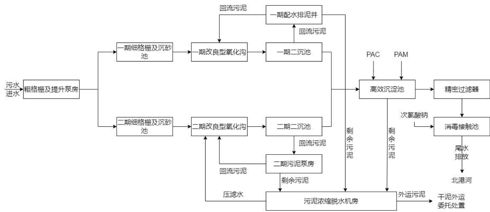
江西洪城水业环保有限公司东乡分公司污水处理工艺流程图
