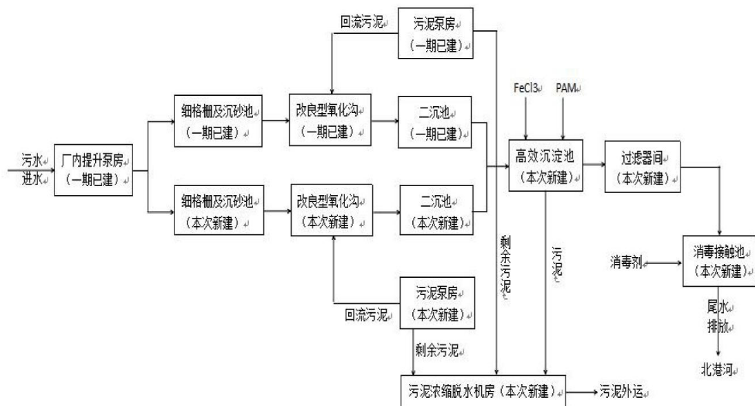
图 2.2-1 东乡区生活污水处理厂工艺流程图
