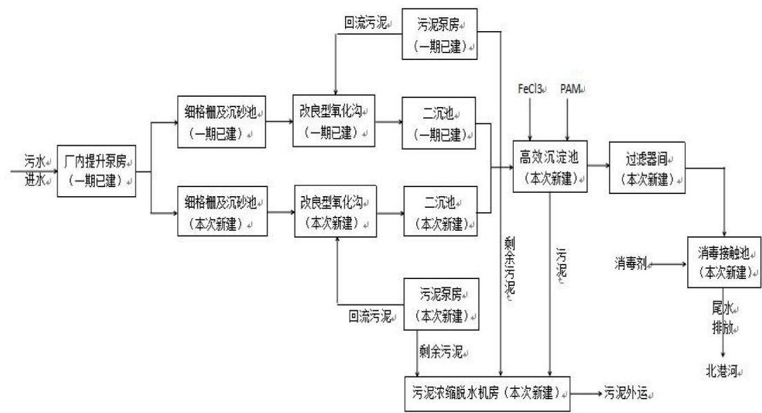
图 3-2 工艺流程图
