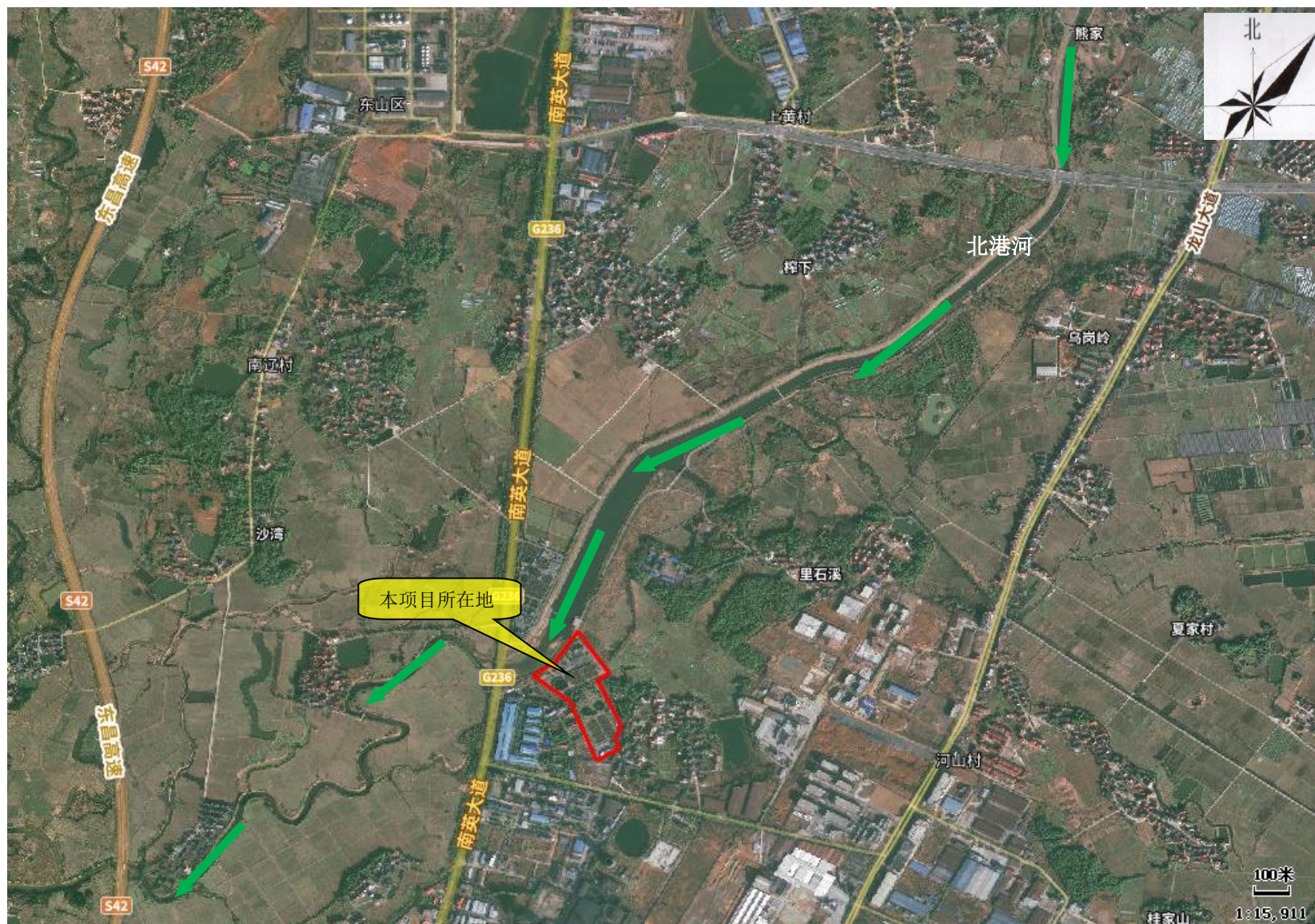
附图4 尾水走向图
