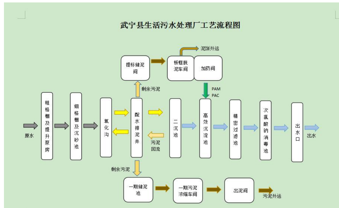
图 1 工艺流程图
